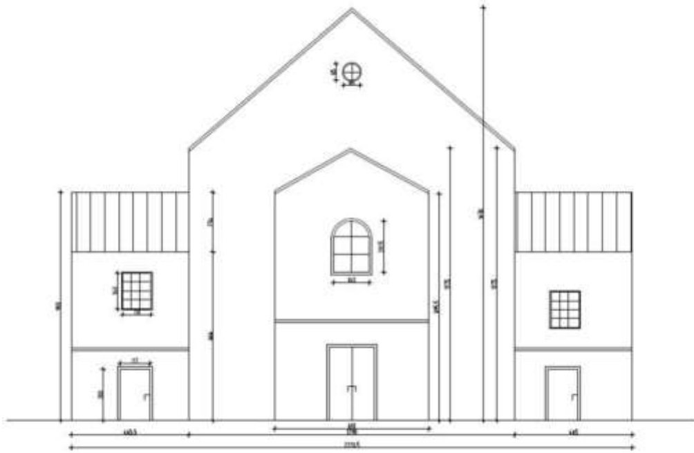
ELEWACJA ZACHODNIA skala 1:100
