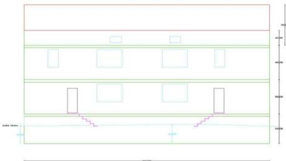
ELEWACJA PÓŁUDNIOWA
